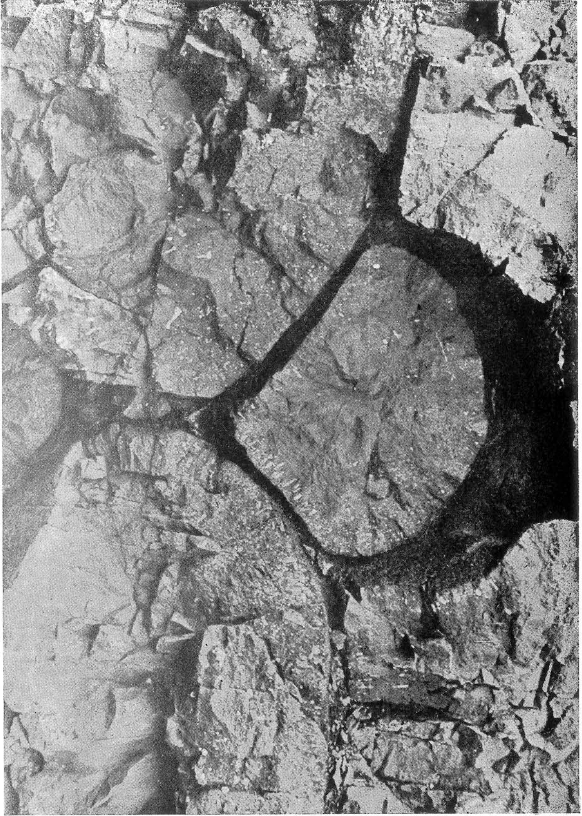
Levha III. Pilov Lavlar, Ankara. Plate III. Pillow Lavas, Ankara.
